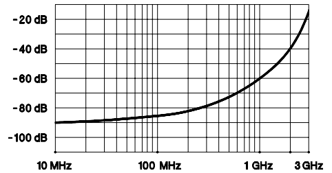
串扰 (75Ω)
