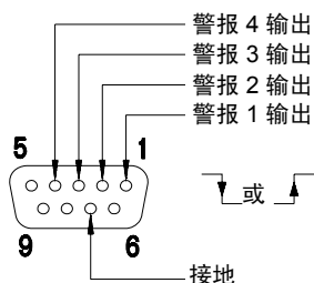
警报连接器
